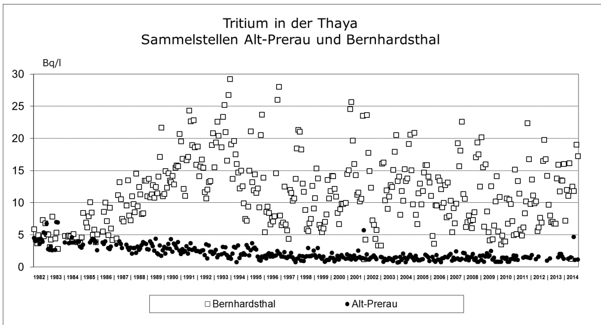
Abb. 4.3.3.: Verlauf der Tritium-Aktivitätskonzentration (Monatswerte) in der Thaya bei Alt-Prerau bzw. bei Bernhardsthal während der Jahre 1982 bis 2014
