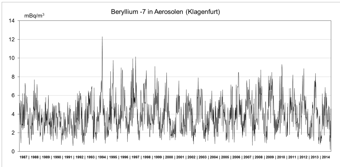
Abb. 4.1.1.: Verlauf der Beryllium-7-Aktivitätskonzentration (Wochenwerte) in Aerosolen während der Jahre 1987 bis 2014 an der Sammelstelle Klagenfurt
