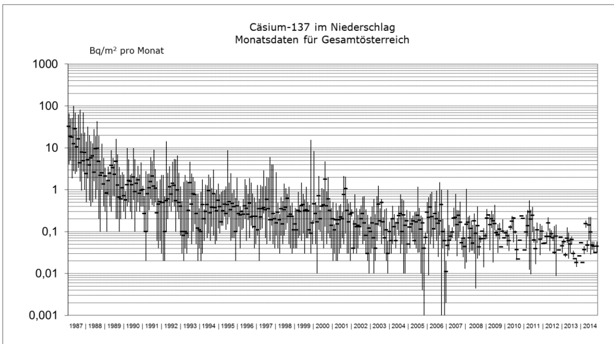
Abb. 4.2.4.: Monatliche Cäsium-137-Flächendeposition während der Jahre 1987 bis 2014 Median- und Extremwerte (log. Skala)
