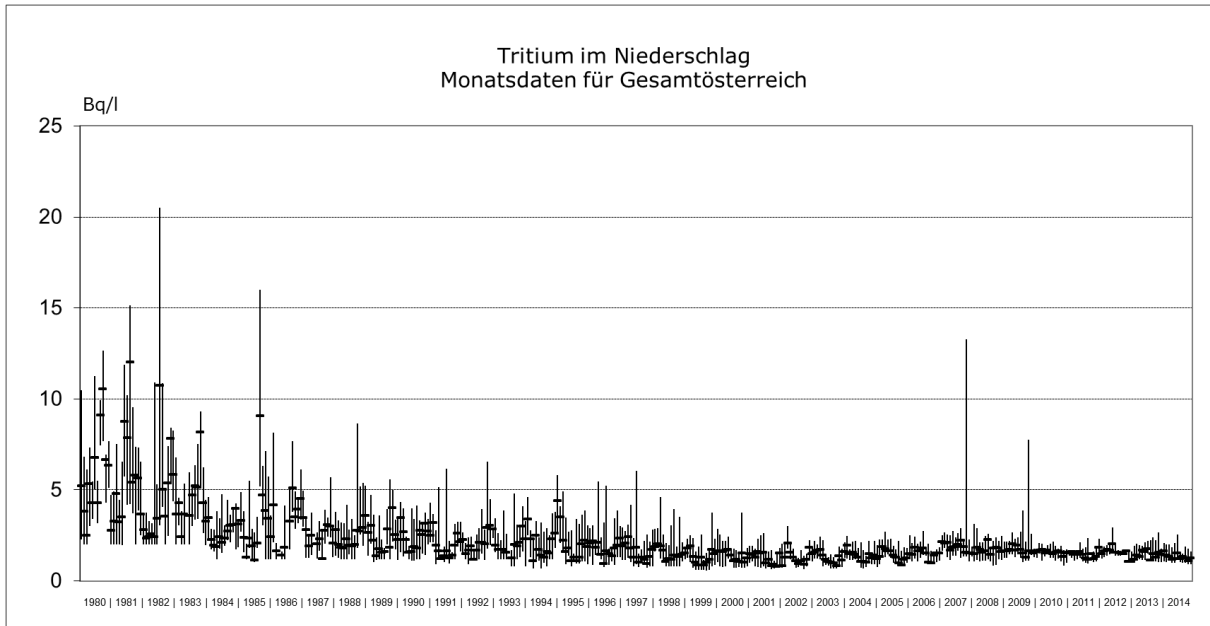
Abb. 4.2.2.: Tritium-Aktivitätskonzentration im Niederschlag während der Jahre 1980 bis 2014 (Median- und Extremwerte)
