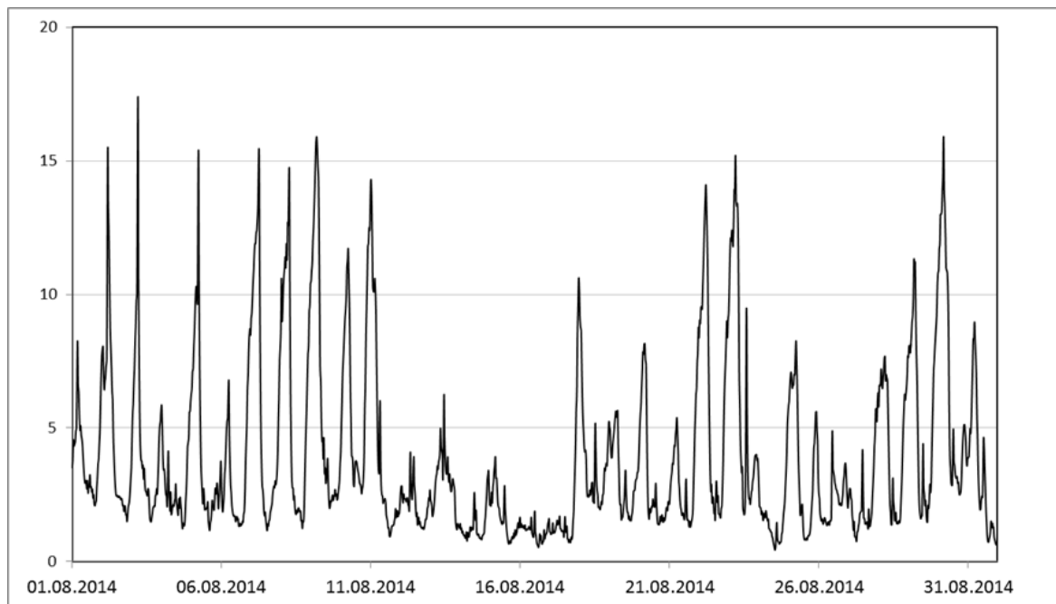
Abb. 3.2.: Verlauf der Radon-222-Konzentration (Stundenwerte) im August 2014 an der Messstelle Leopoldschlag
