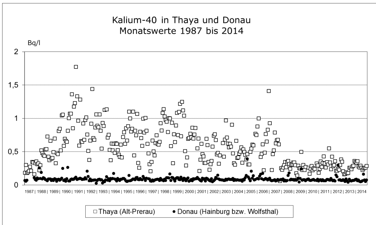
Abb. 4.3.1.: Verlauf der Kalium-40-Aktivitätskonzentration in der Thaya bei Alt-Prerau und in der Donau bei Hainburg bzw. Wolfsthal während der Jahre 1987 bis 2014
