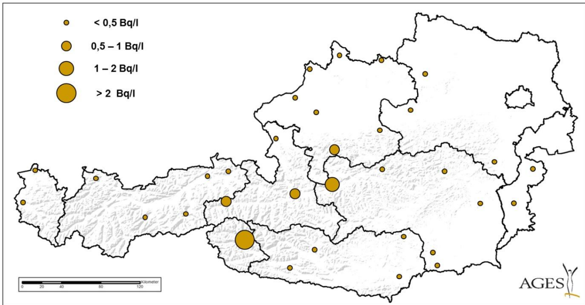
Abb. 4.6.1.1.: Regionale Verteilung der Cäsium-137-Kontamination von Rohmilch in Österreich für die Jahre 2013 und 2014
