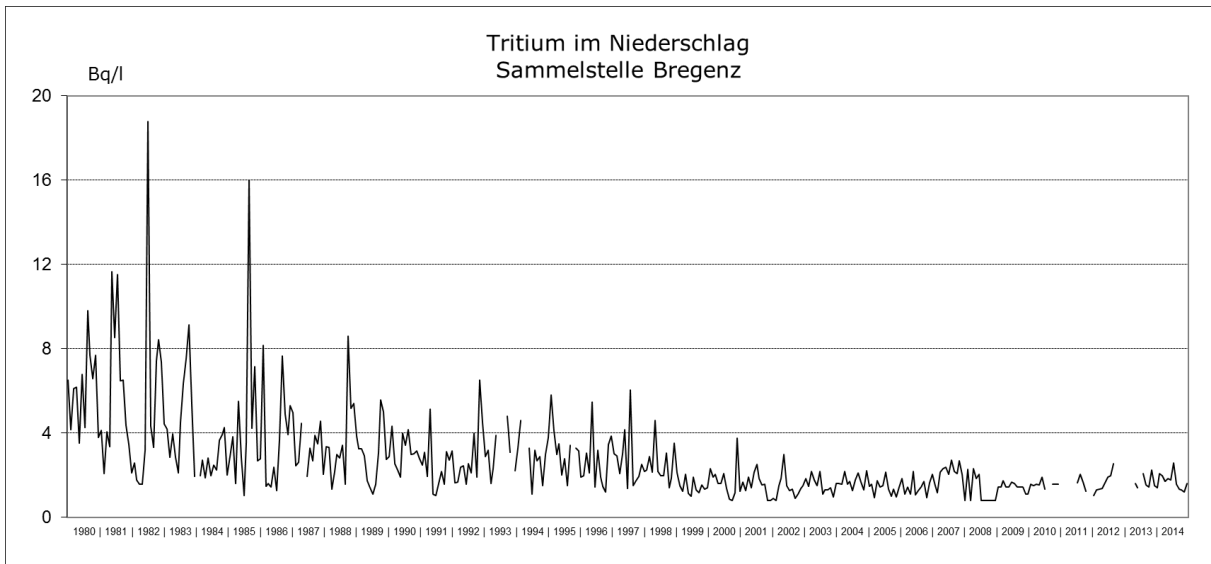
Abb. 4.2.3.: Verlauf der Tritium-Aktivitätskonzentration (Monatswerte) im Niederschlag während der Jahre 1980 bis 2014 für die Sammelstelle Bregenz
