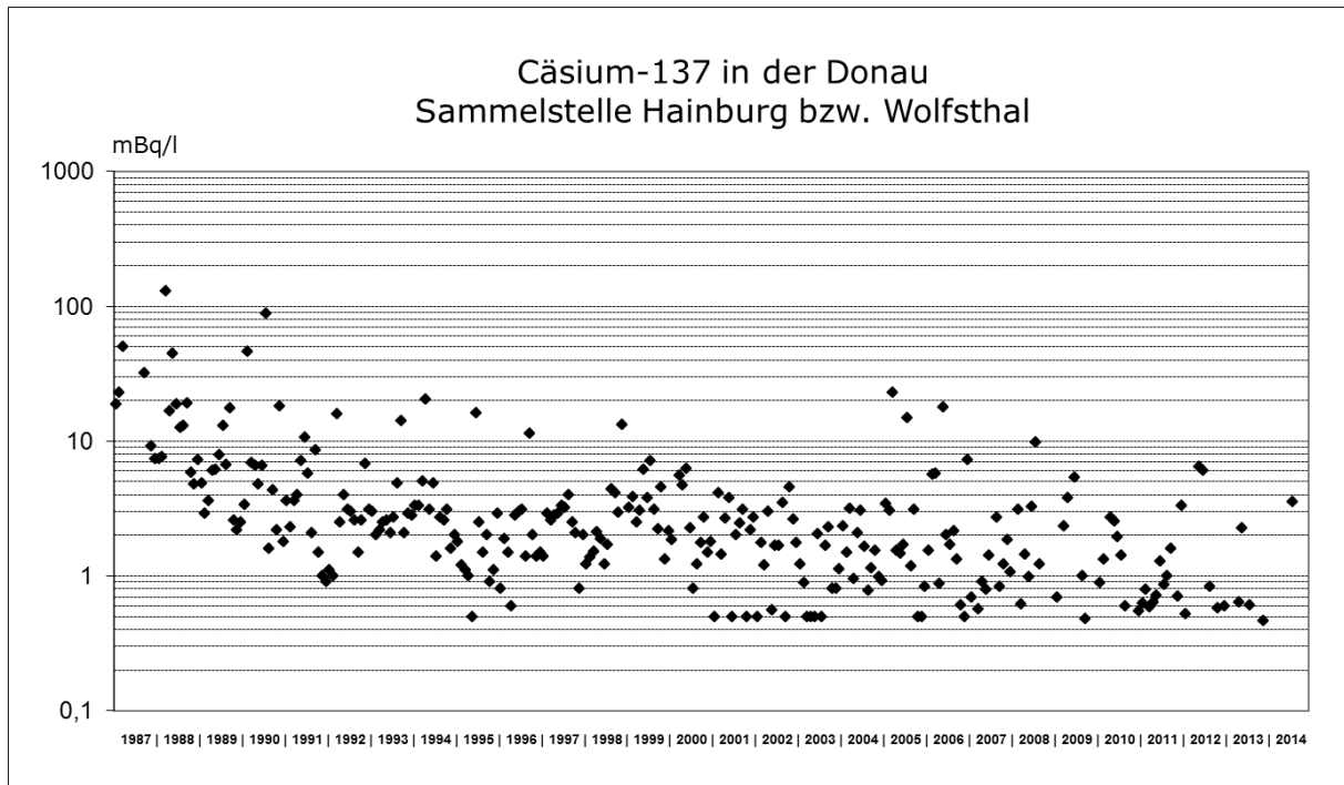
Abb. 4.3.5.: Verlauf der Cäsium-137-Aktivitätskonzentration in der Donau bei Hainburg bzw. Wolfsthal während der Jahre 1987 bis 2014 (log. Skala)
