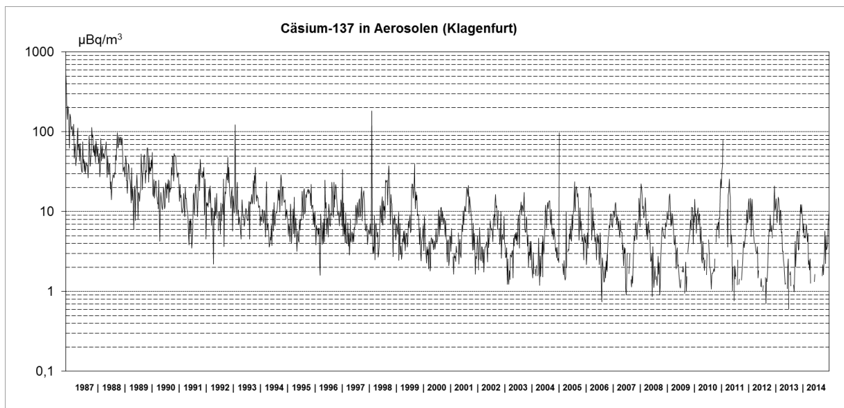
Abb. 4.1.2.: Verlauf der Cäsium-137-Aktivitätskonzentration (Wochenwerte) in Aerosolen während der Jahre 1987 bis 2014 an der Sammelstelle Klagenfurt (log. Skala)
