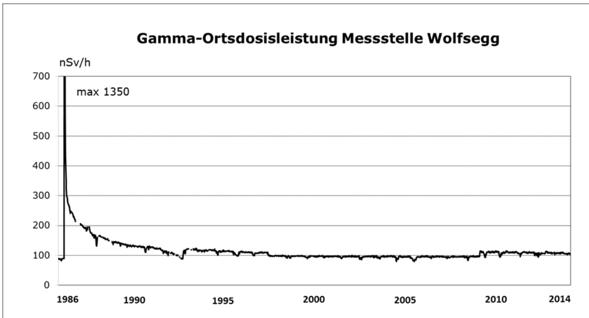
Abb. 3.1.: Verlauf der Ortsdosisleistung (Wochenmittelwerte) während der Jahre 1986 bis 2014 an der Messstelle Wolfsegg (OÖ)
