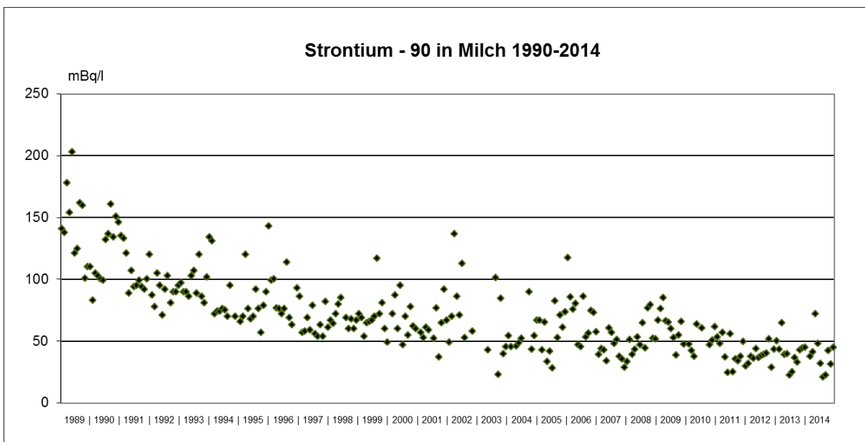
Abb. 4.6.1.4.: Strontium-90-Kontamination von Rohmilch aus Wiener Molkereien bzw. der Molkerei Baden (bis 1999) und Milch aus dem Handel (ab 2000)
