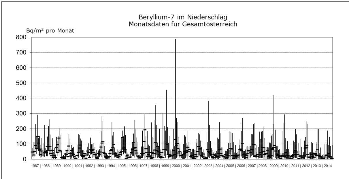
Abb. 4.2.1.: Monatliche Beryllium-7-Flächendeposition während der Jahre 1987 bis 2014 (Median- und Extremwerte)
