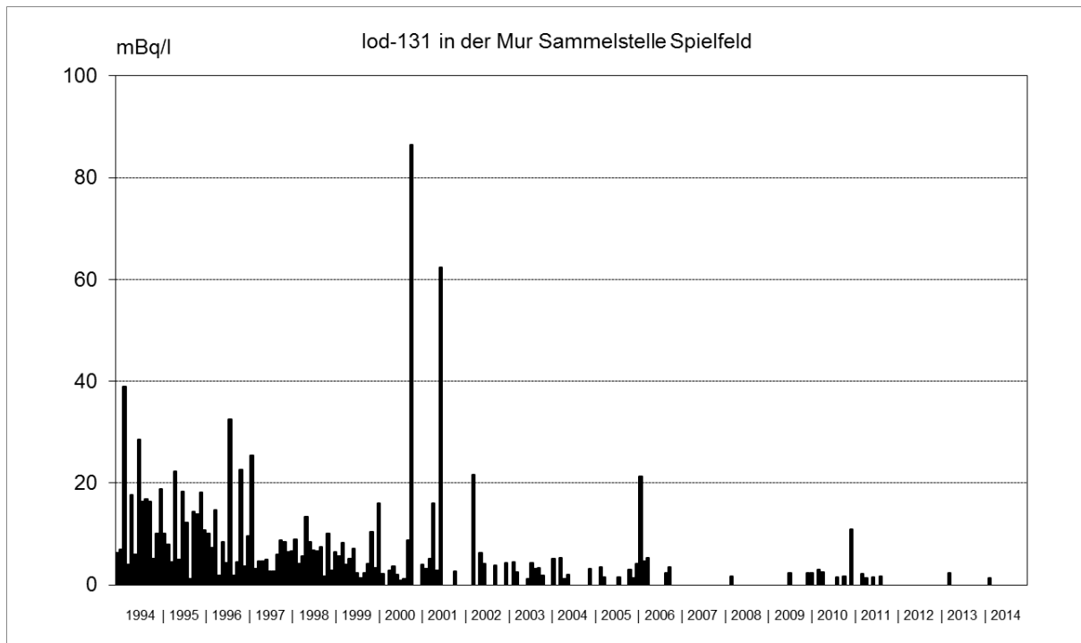
Abb. 4.3.6.: Verlauf der Iod-131-Konzentration (Monatswerte) in der Mur bei Spielfeld während der Jahre 1994 bis 2014
