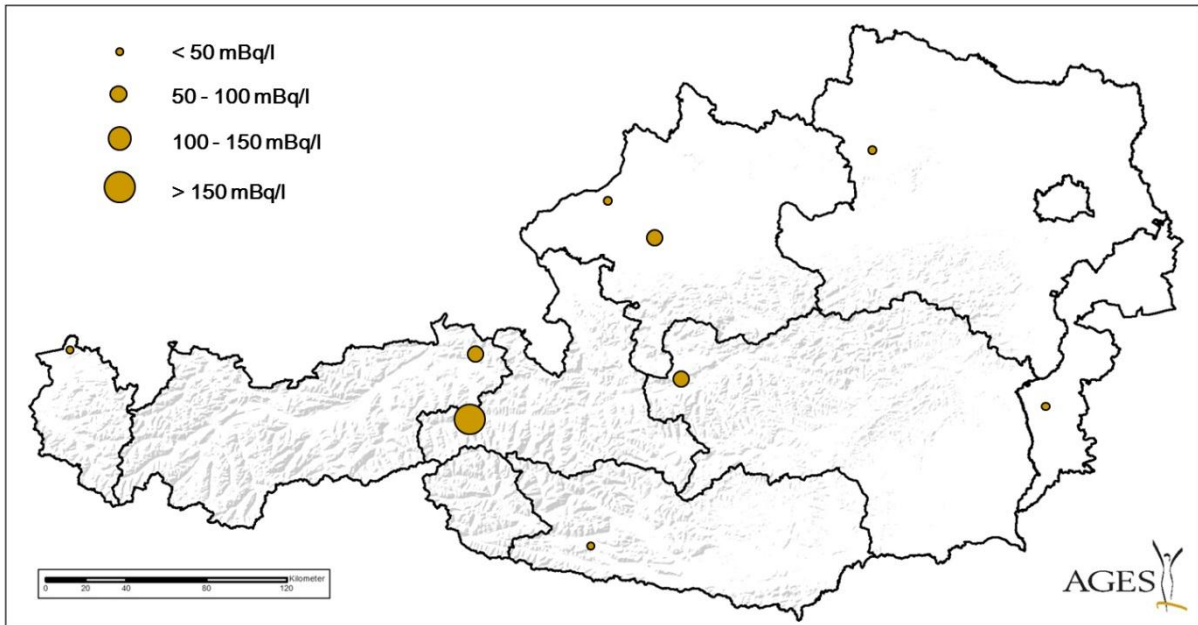
Abb. 4.6.1.3.: Regionale Verteilung der Strontium-90-Kontamination von Rohmilch in Österreich für die Jahre 2013 und 2014
