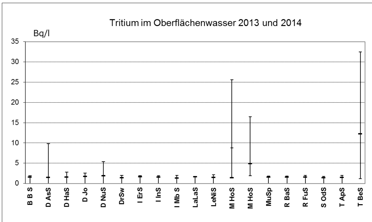
Abb. 4.3.2.: Mittelwerte (Median) sowie minimale und maximale Werte der Tritium-Aktivitätskonzentration in Oberflächenwasser für die Jahre 2013 und 2014
