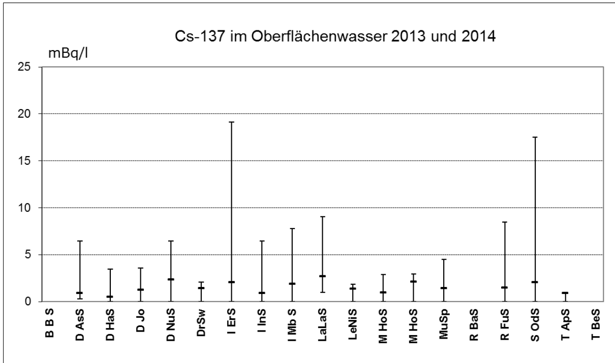
Abb. 4.3.4.: Jahresmittelwerte sowie minimale und maximale Werte der Cäsium-137-Aktivitätskonzentration in Oberflächenwasser für die Jahre 2013 und 2014
